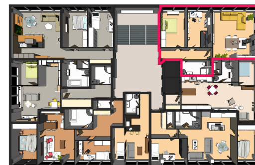
Půdorys patra
